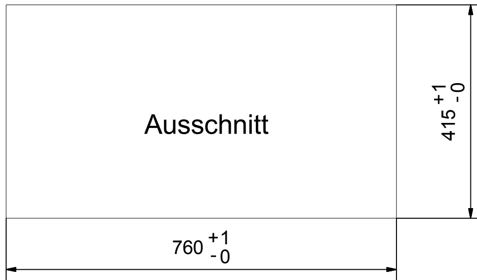
Konstruktionszeichnung 0002-110777
