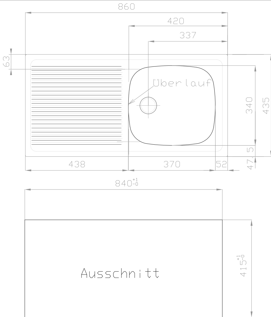
Konstruktionszeichnung S13. 1. 1850
